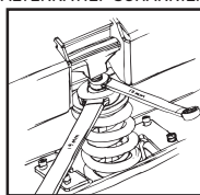
ALTERNATIEF SCHARNIER
