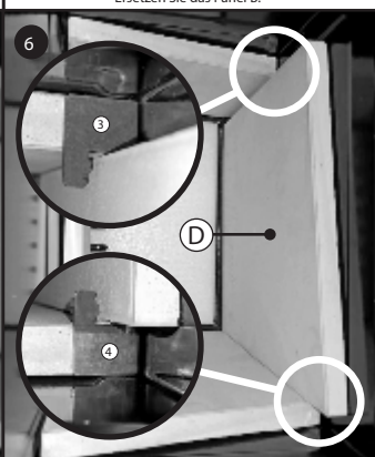
Tauschen Sie Panel D aus. Halterungen 3 und 4 hinzufügen.
