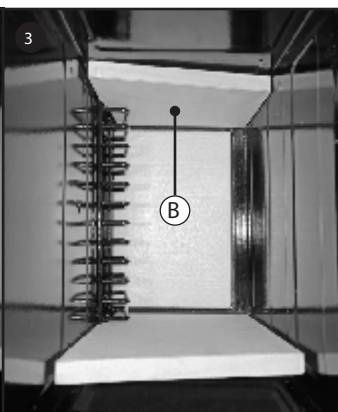
Ersetzen Sie das Panel B.
