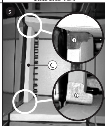
Fügen Sie Klammer 1 und 2 hinzu.
